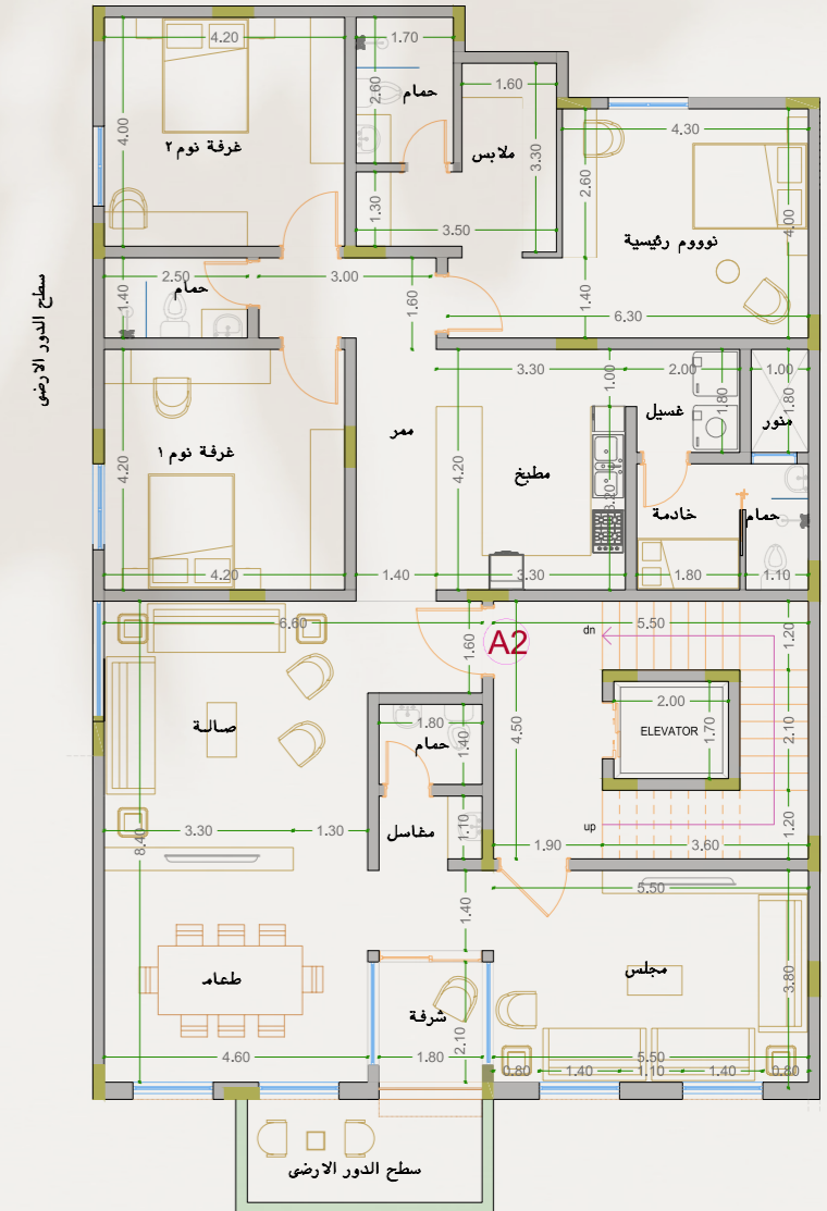
الدور الأول First Floor
